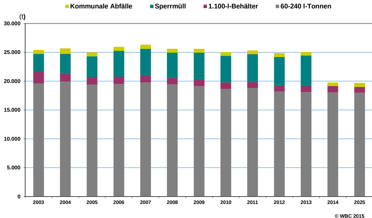
Abb. 19: Abfälle zur Beseitigung aus den kommunalen Erfassungssystemen im Kreis Coesfeld sowie Prognose für 2025 in Gewichtstonnen
