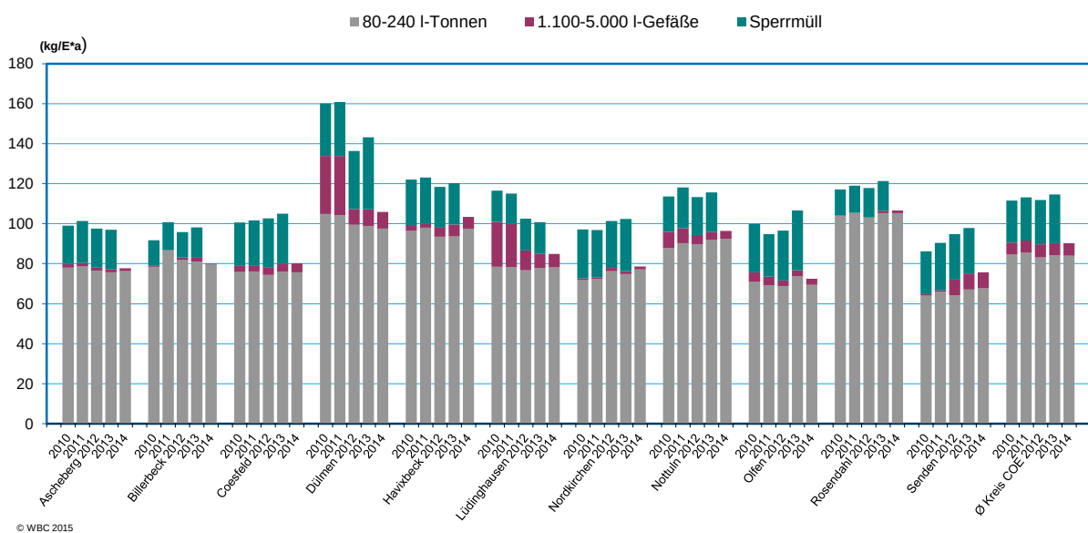
Abb. 20: Abfälle zur Beseitigung 2010 - 2014 in den Städten und Gemeinden des Kreises Coesfeld in kg/Ea
